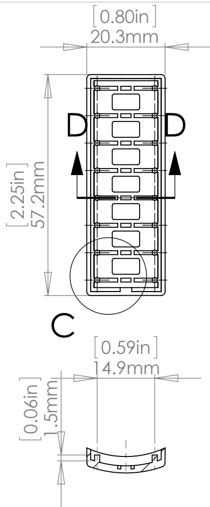
SECTION D-D
